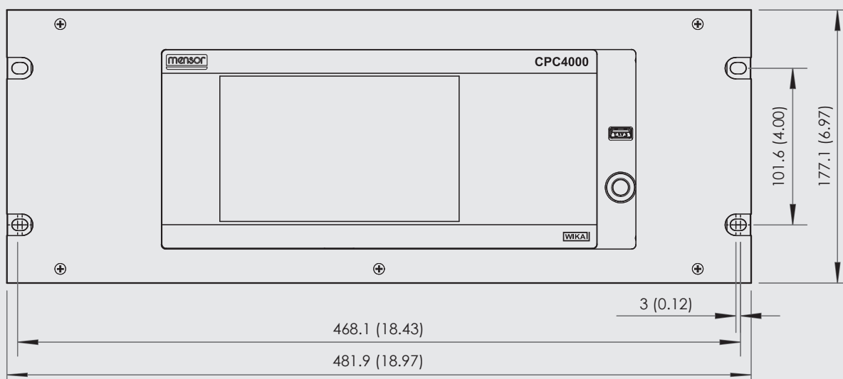
Kit per montaggio a rack da 19", vista frontale
